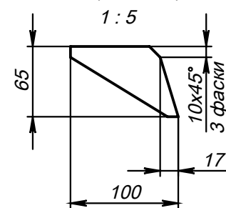
Поз.4 (Косынка)
