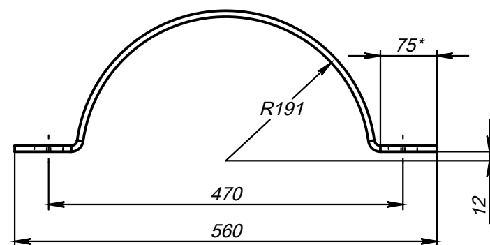
Поз.3 (Полухомут)
